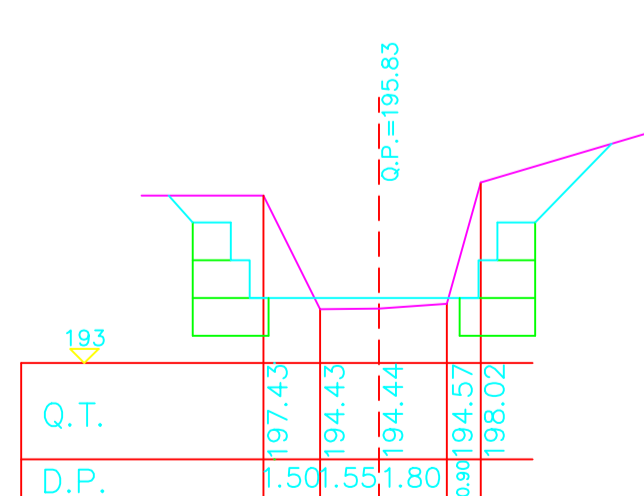
Sez.39
