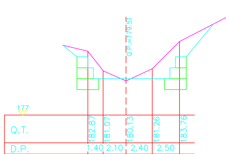
Sez.33
