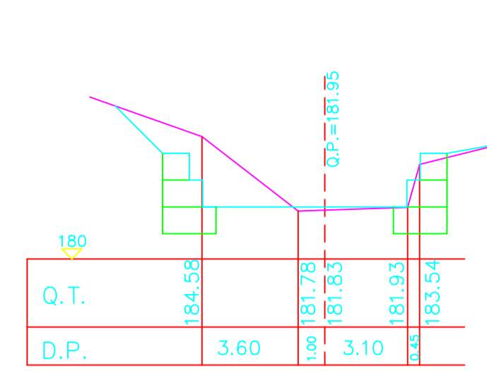
Sez.34
