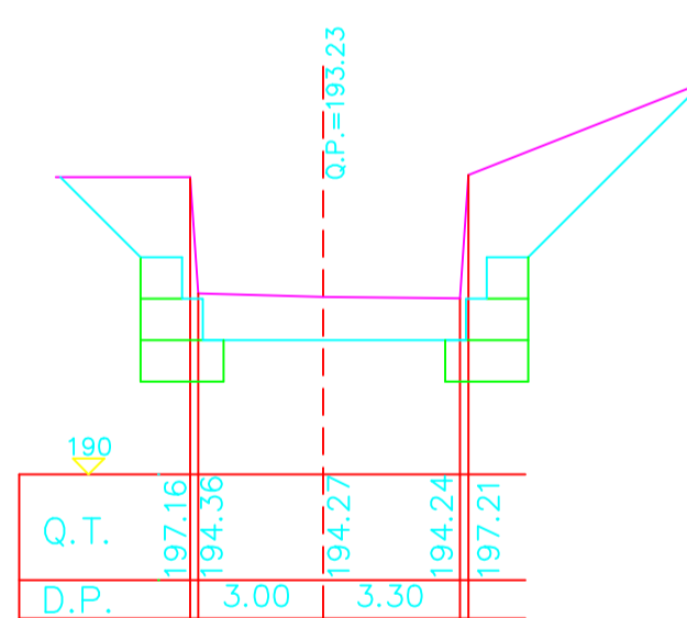
Sez.38
