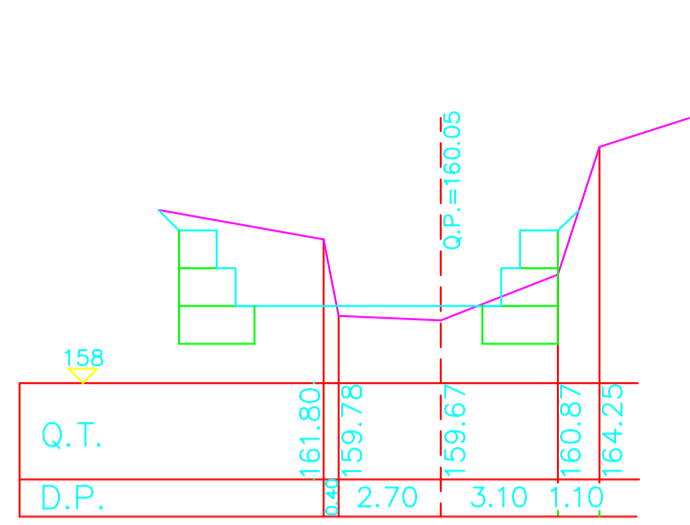
Sez.29
