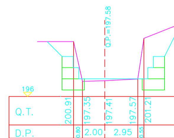
Sez.40
