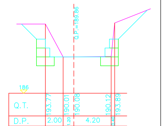
Sez.37
