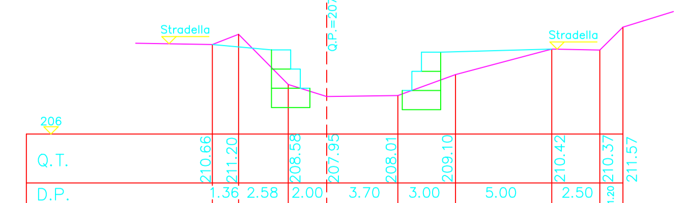
Sez.43
