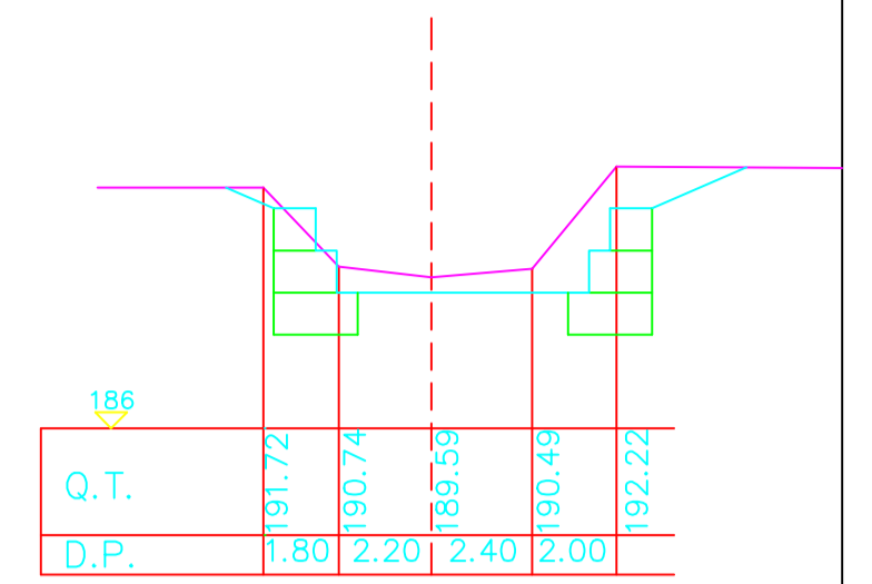
Sez.36
