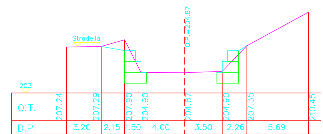
Sez.42
