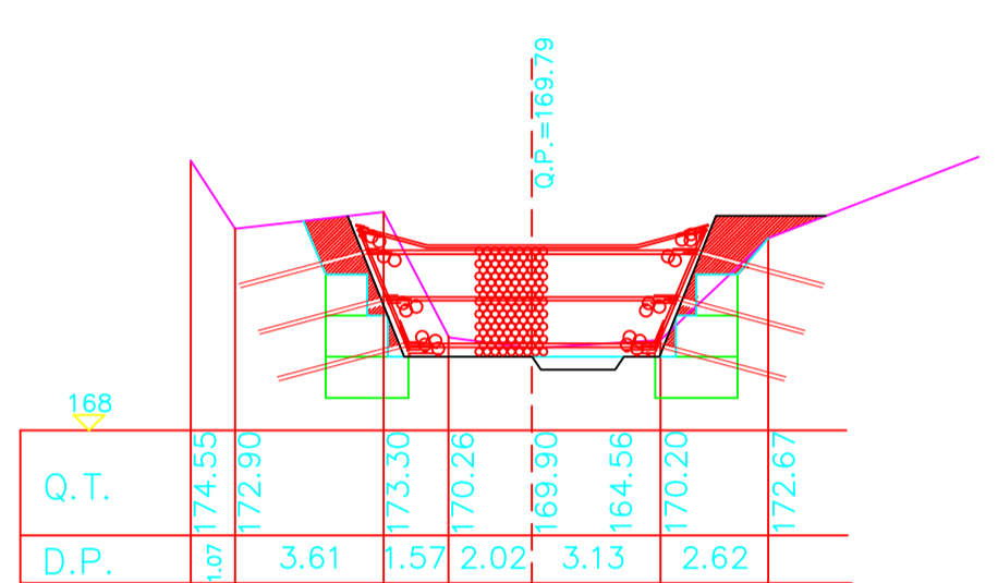
Sez.31t
