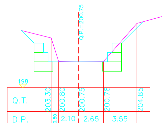
Sez.41
