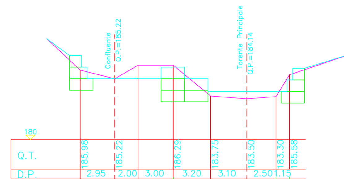
Sez.35
