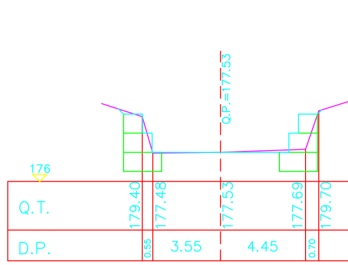
Sez.32
